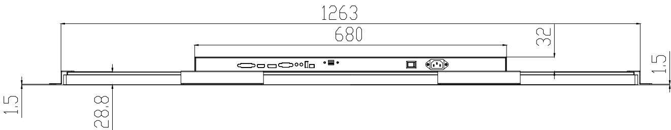
СХЕМА ДИСПЛЕЯ (ВИД СНИЗУ)
